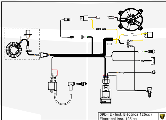
09b-IE - Inst. Eléctrica 125cc / Electrical Inst. 125 cc
